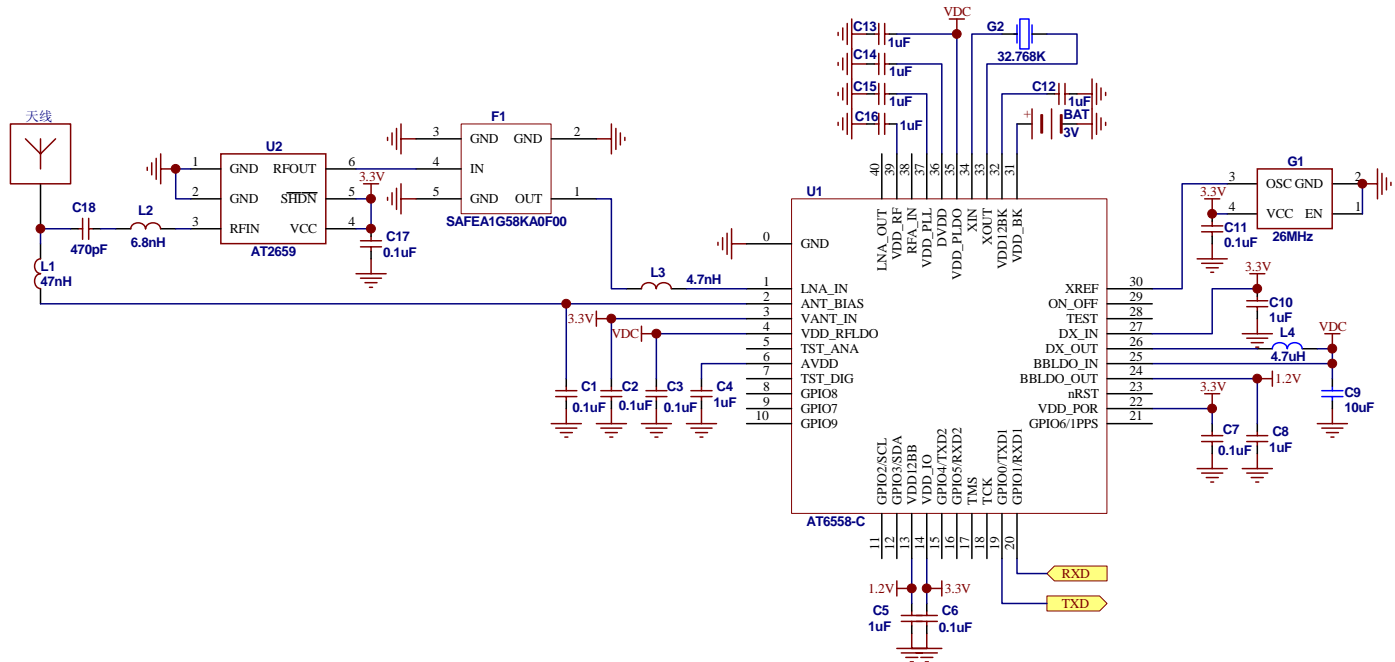
AT6558-C应用线路图
